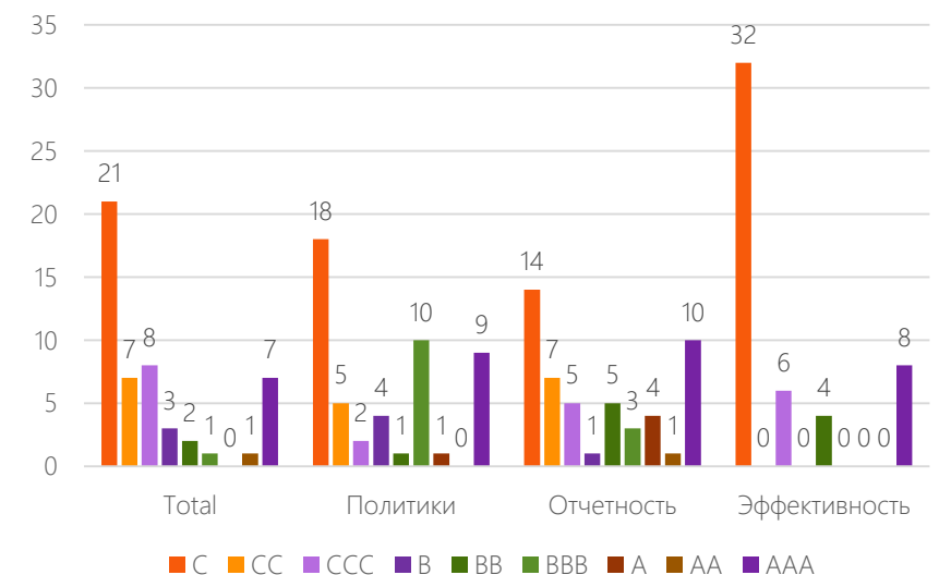
Распределение участников по блоку Возобновляемая энергия
